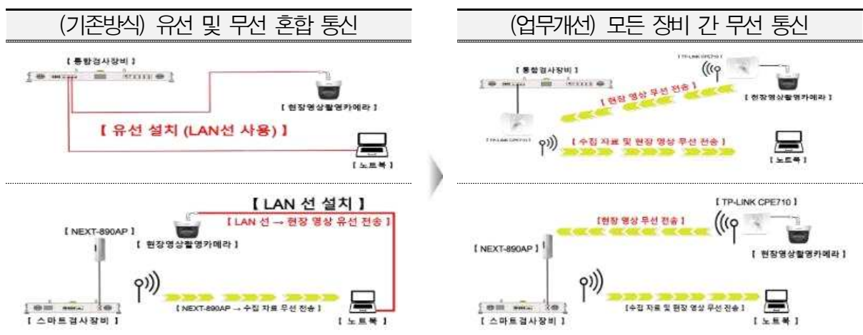
[그림 1] 무인단속검사 장비 연결 개념도
